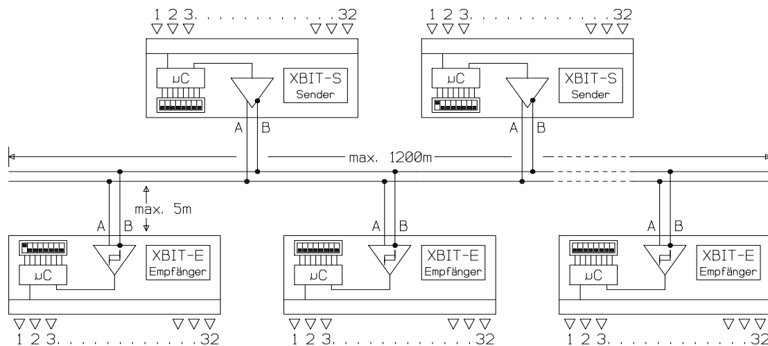
XBIT-S Sendeplatine
